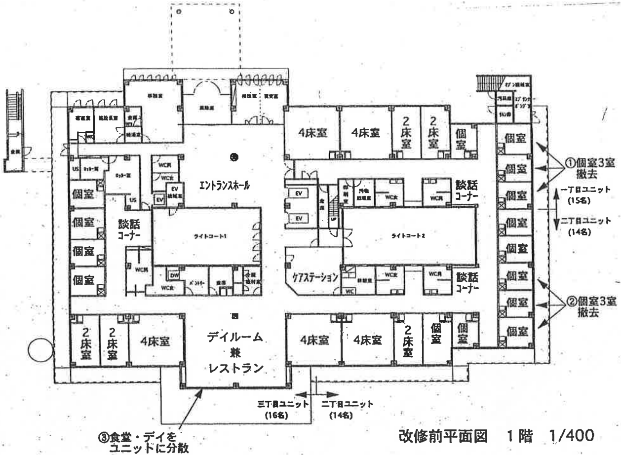
図1：改修前後平面図 1/400 1階
