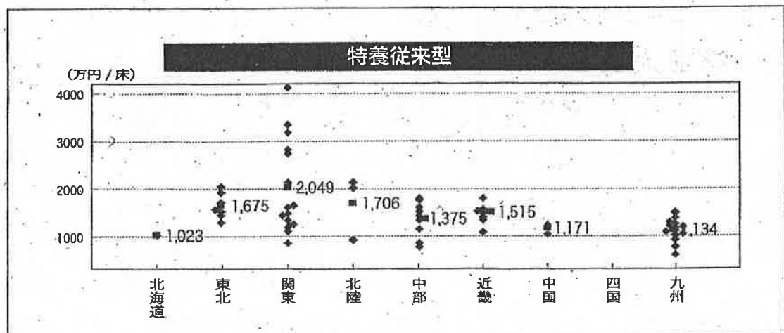
図表 2-7 建設地域別みた1床あたり建設単価
