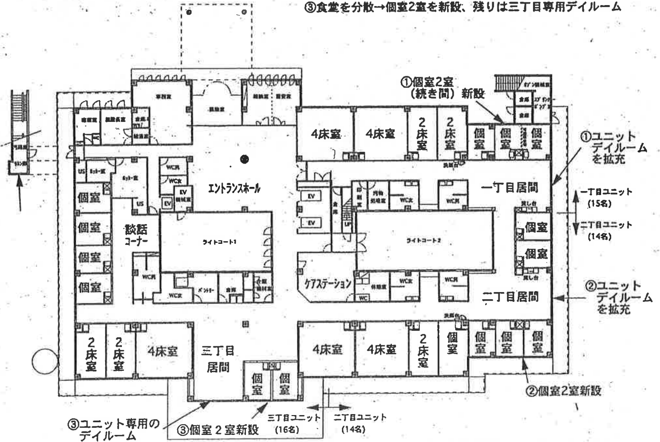
改修後平面図 1階 1/400
