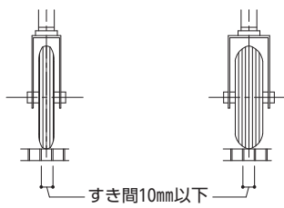
【図3.1】車椅子の前輪が落下しない配慮
