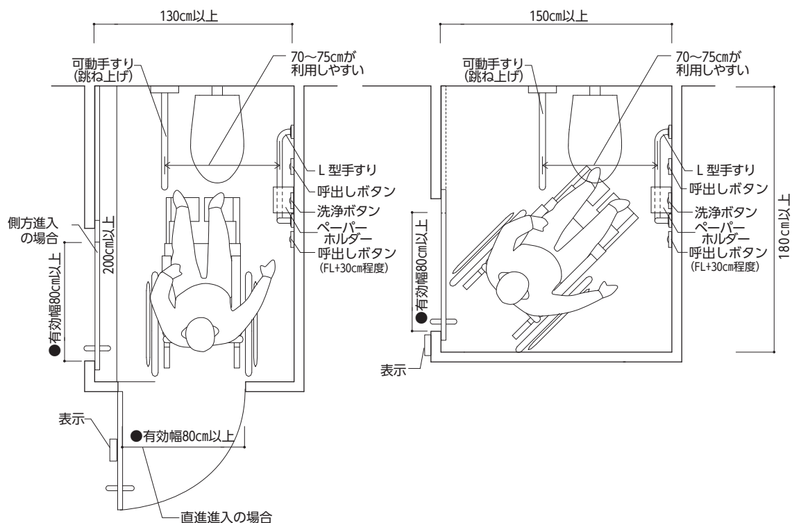
【図2.1】 車椅子使用者も利用できる広めの便房の例
