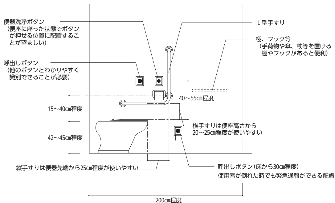
【図2.4】 ボタンの配置例
