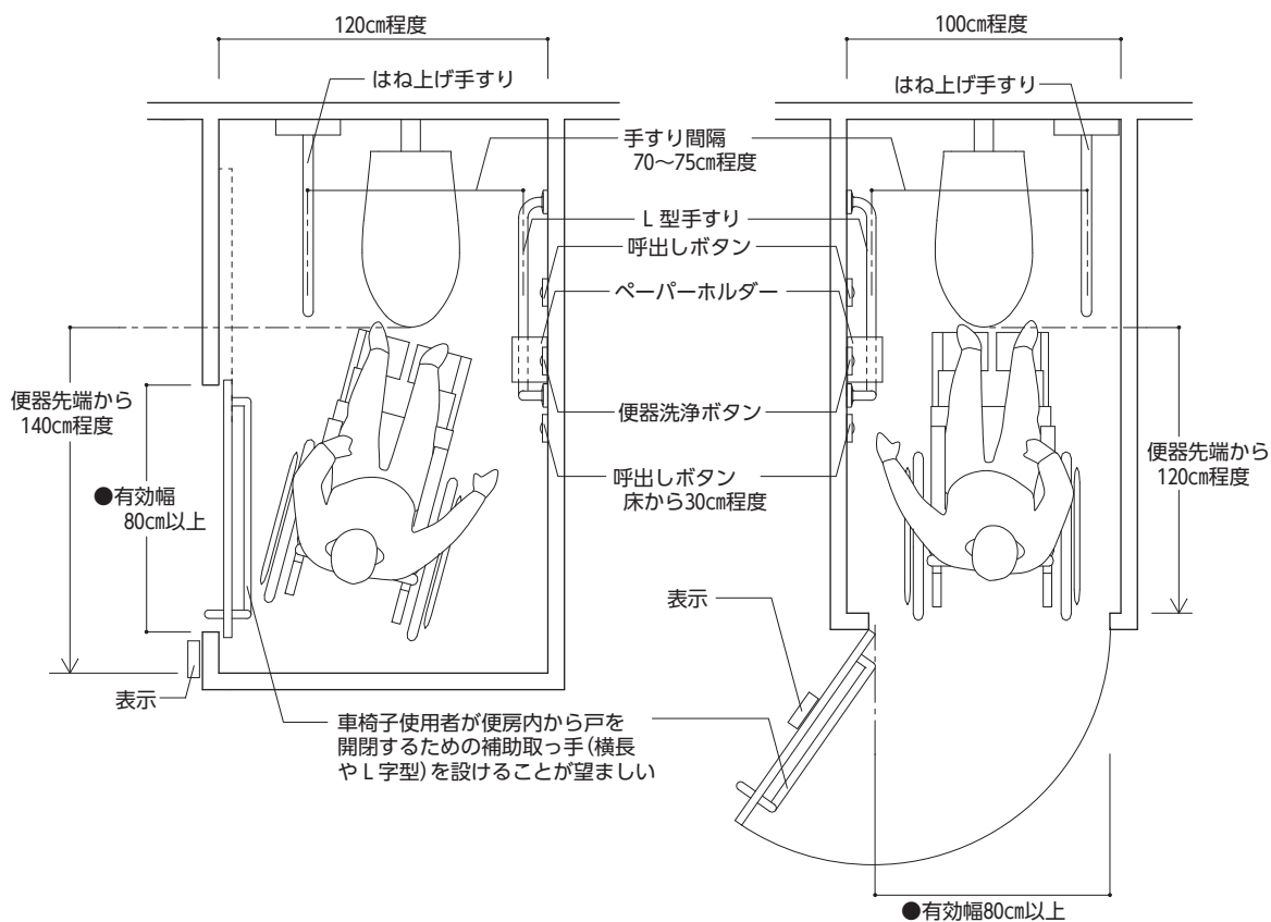
【図2.2】 既存建築物の改修等の構造上やむを得ない場合等の例
