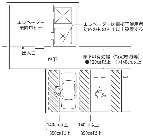
【図11.2】 地下駐車場の整備例
