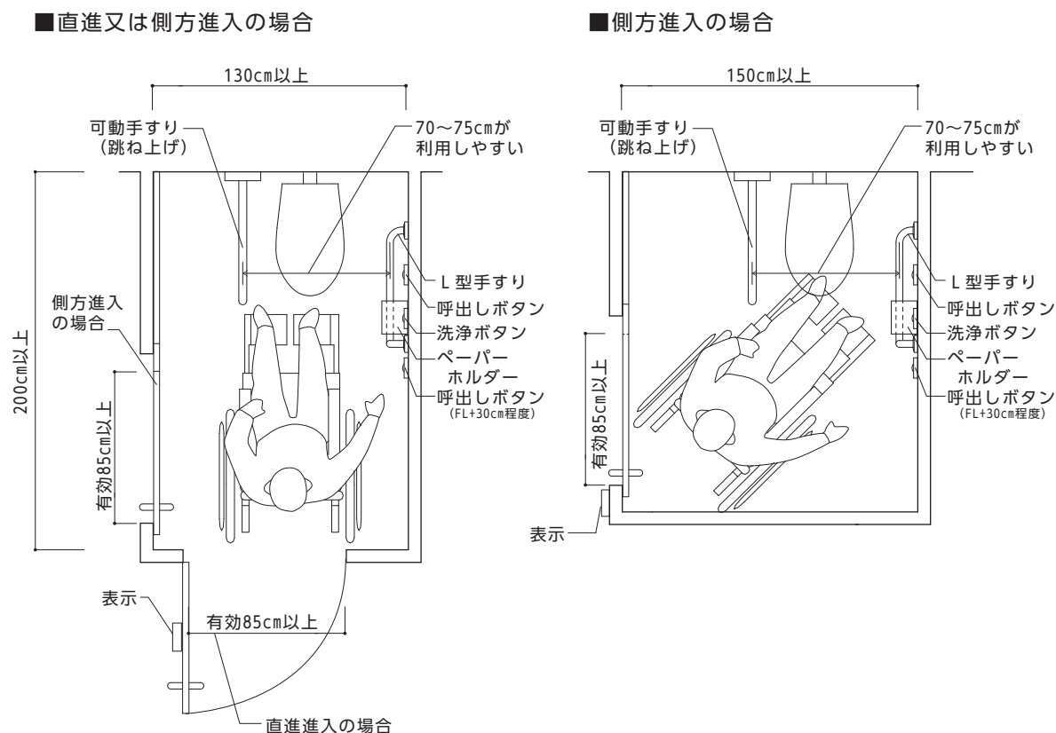
【図8.3】車椅子利用者も利用できる広めの便房の例
