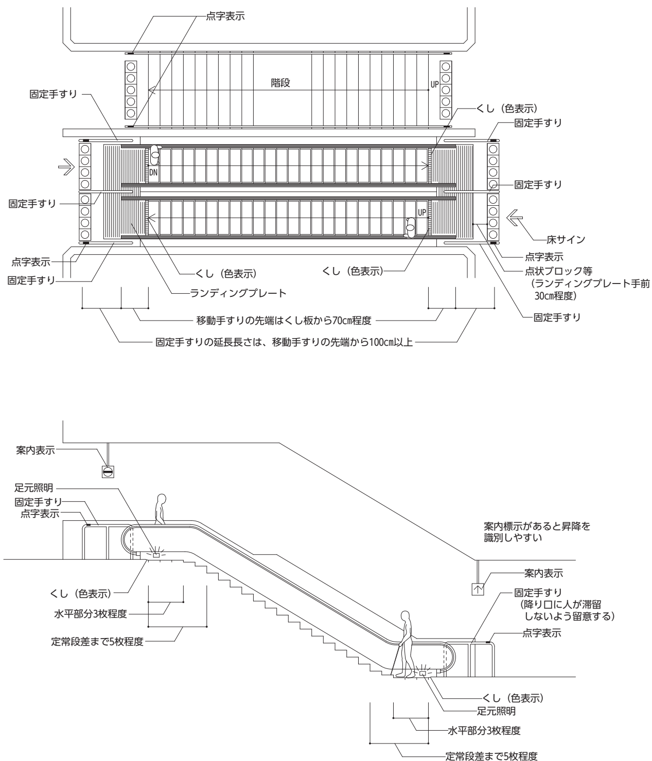
【図7.4】 エスカレーターの場合
