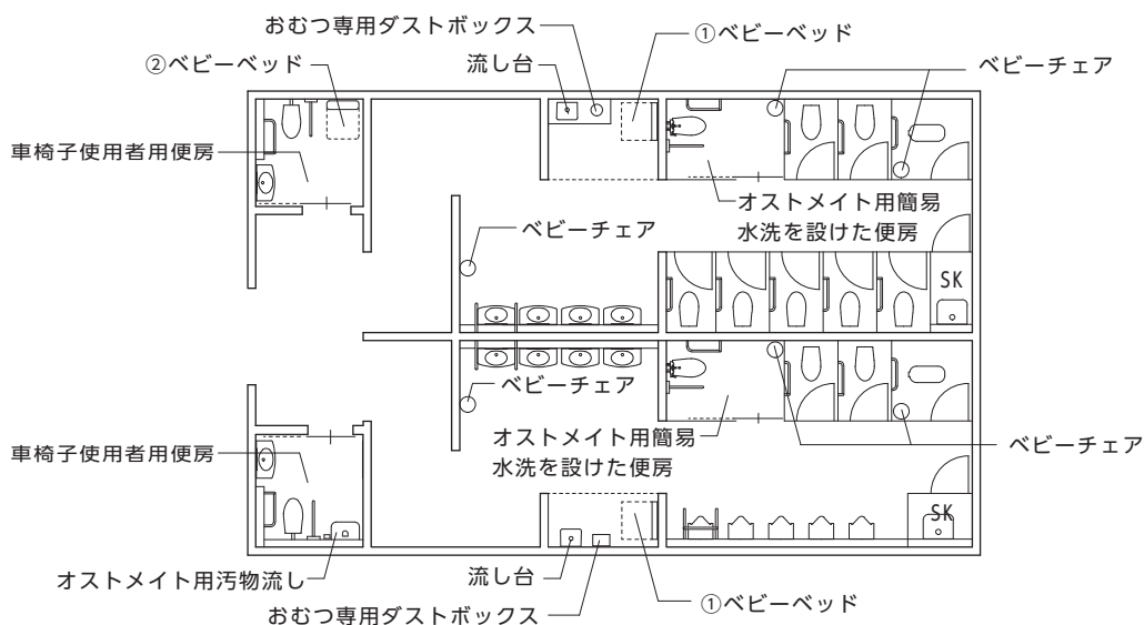
【図18.3】 ベビーチェア・ベビーベッドのレイアウト例
