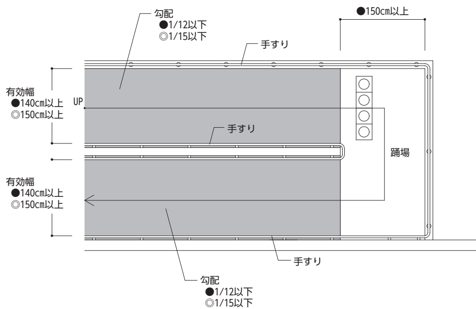
【図5.3】 踊場の設置例
