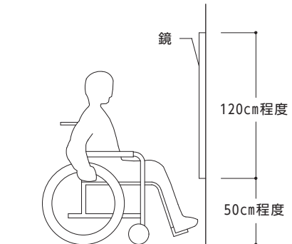
【図8.15】 便房内の身づくろい用鏡の高さの例
