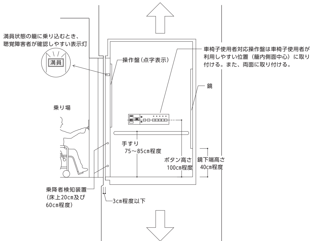
【図6.3】 籠内の断面図
