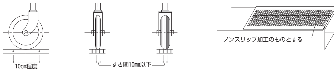
【図12.2】 敷地内の通路
