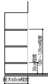
【図10.9】 カウンターの例
