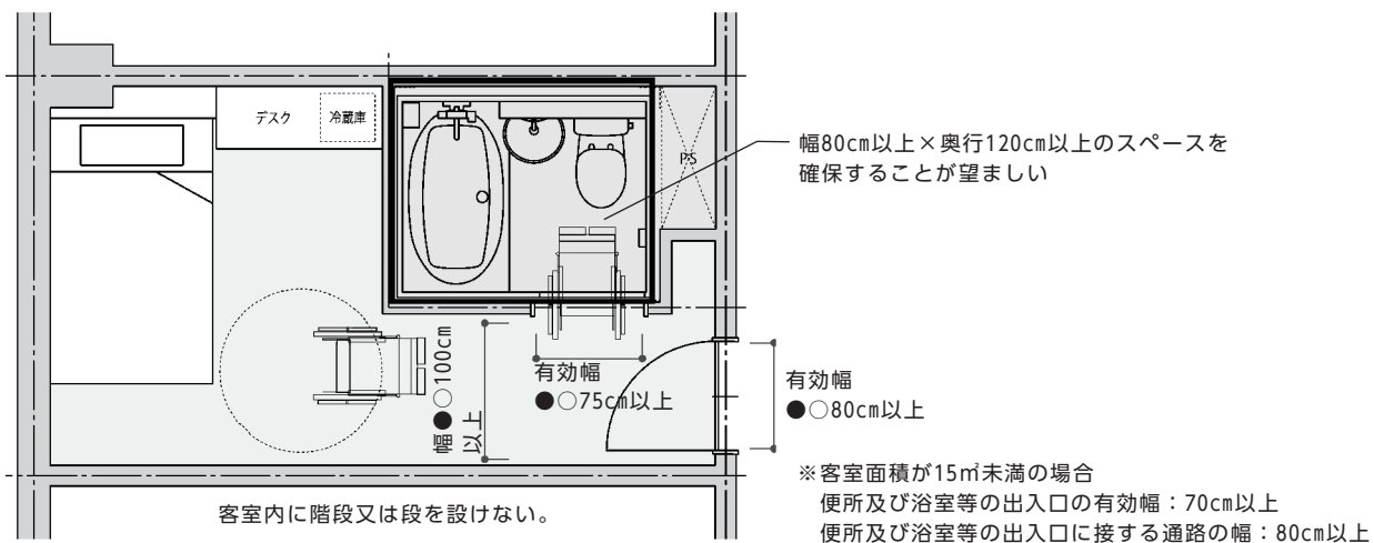
【図10.6】一般客室の例（客室面積15㎡）
