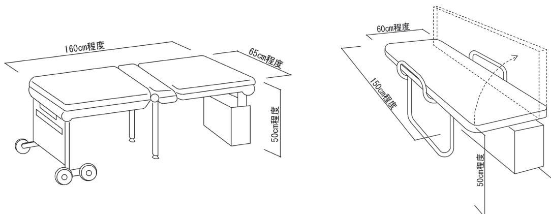
【図8.13】据置型の折り畳み式介助用ベッドの例（幼児～大人まで：折り畳み収納型）
