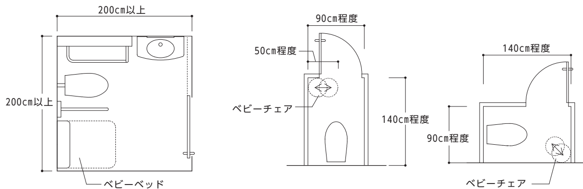
【図18.6】 便房内にはベビーベッド、ベビーチェアを設ける例
