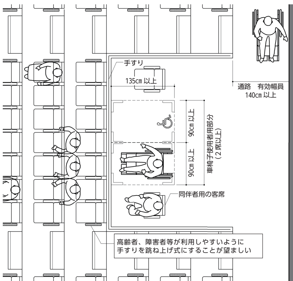
【図11.1】観覧席・客席の例
