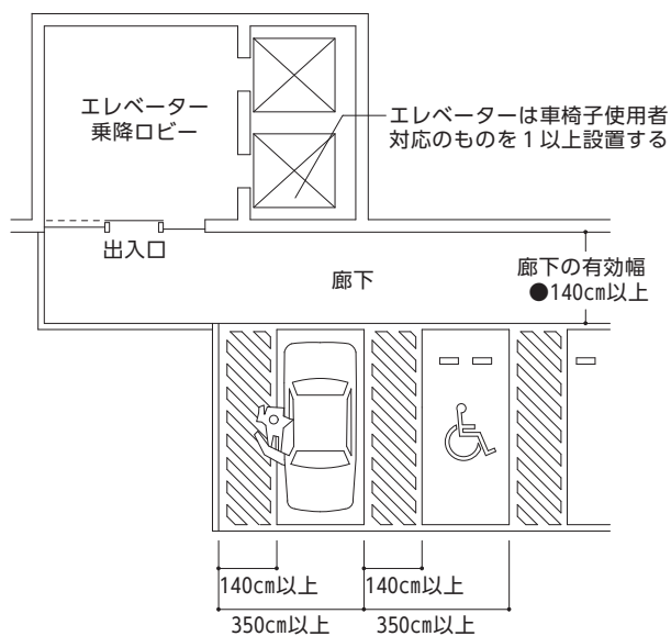
【図13.2】地下駐車場の整備例
