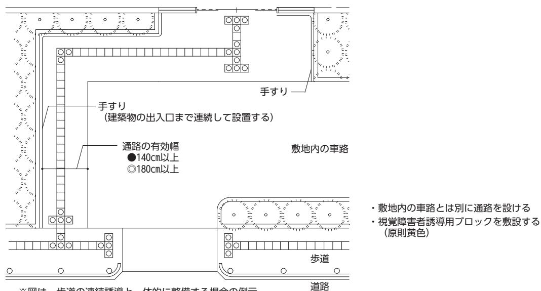
【図12.2】 敷地内の通路
