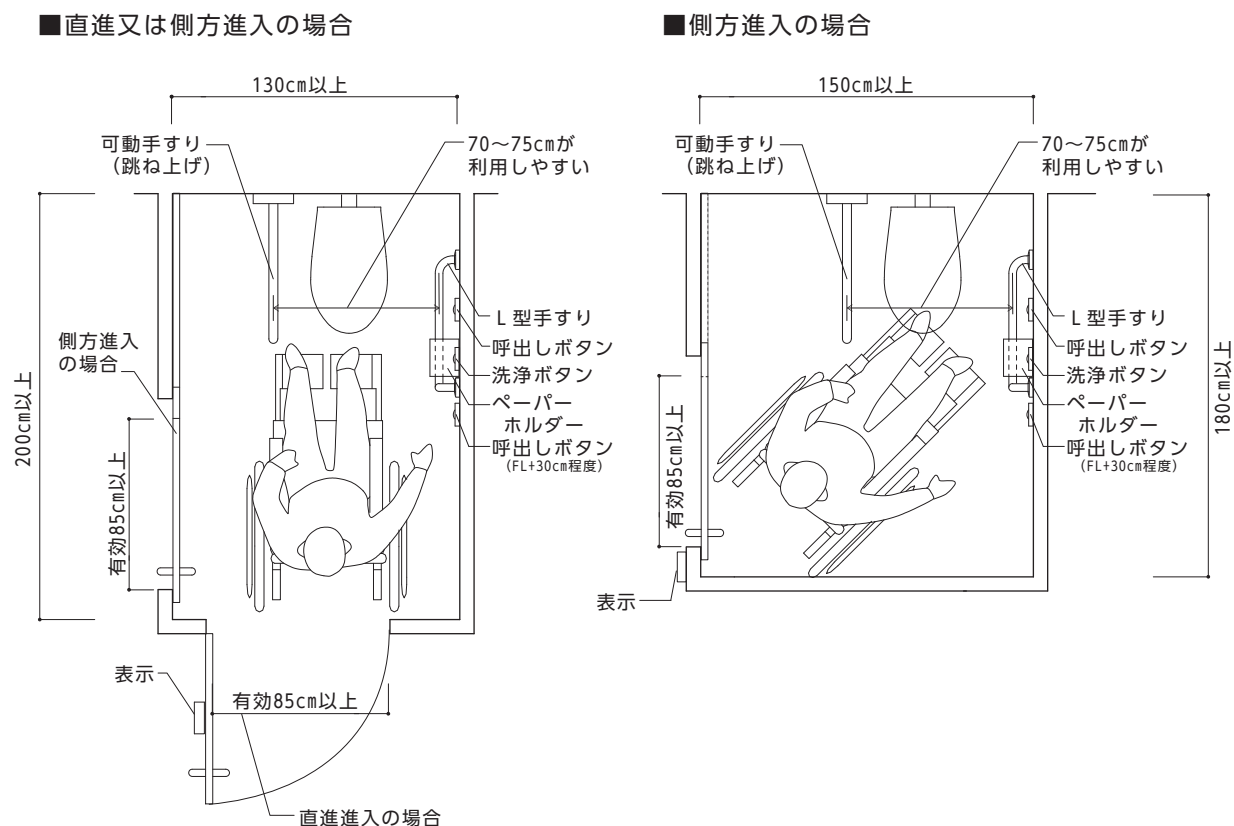
【図8.4】車椅子利用者も利用できる広めの便房の例
