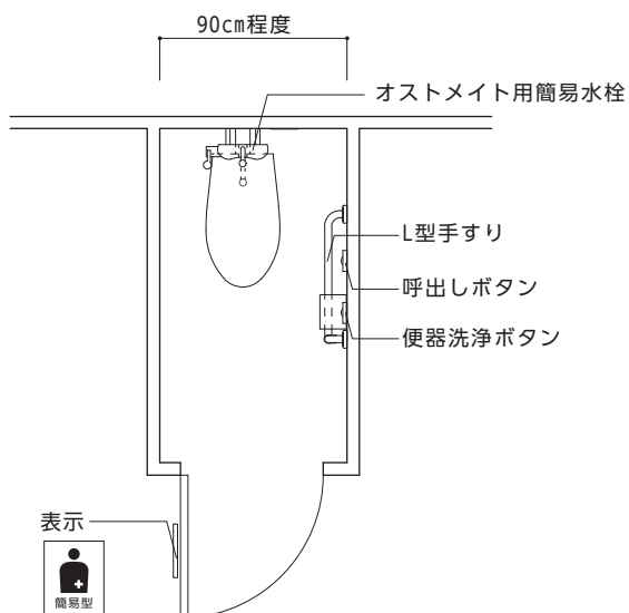
【図8.16】 オストメイト用簡易水栓を設けた例
